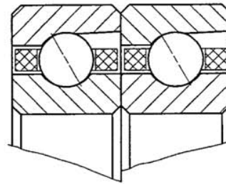
T—TYPE DUPLEX TANDEM (DT)
